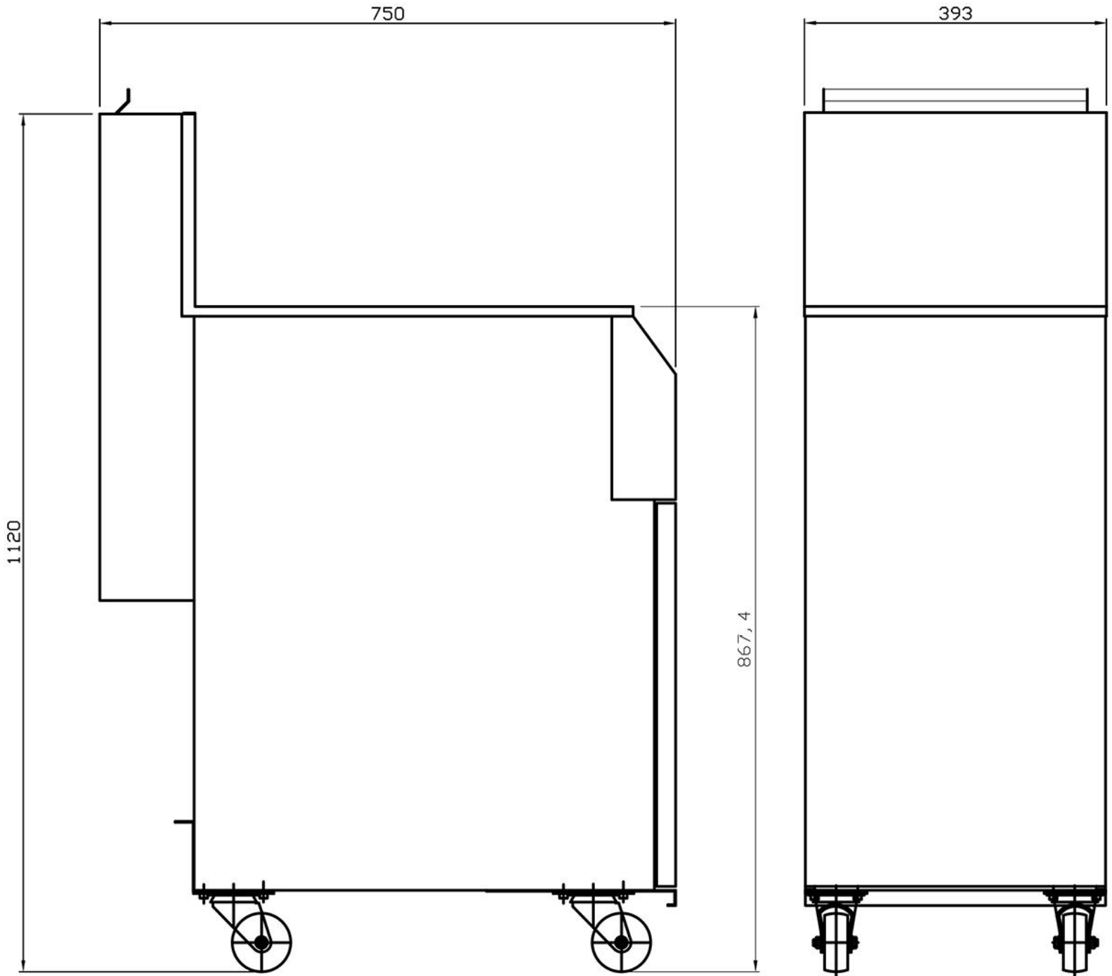
DIMENSIONAL DA FRITADEIRA JJ 18-22 G/E
