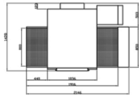
DIMENSIONAL FORNO JJ 00-104 ESTE EQUIPAMENTO PODERA SER SUBROFISTO EM ATÉ 2 UNIDADES
